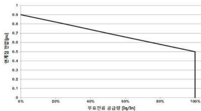
[고장발생 후 무효전류 공급능력]
