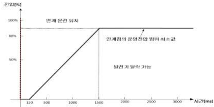
[순시전압저하시 연계운전 유지성능]
